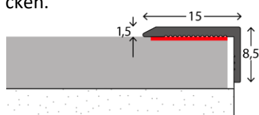
Abb. Eckprofil
