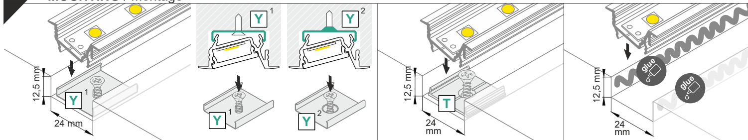
Y flexible mounting plate Einbaumaß mit Halter Y
